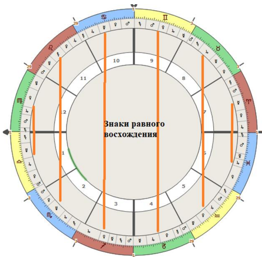
Рисунок 17. Знаки равного восхождения или контрантисы.
